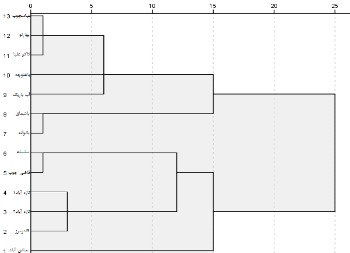
شکل ۴ - درختواره خوشه بندی روستاهای نمونه بر اساس شدت خشکسالی در شهرستان های قروه و دهگلان طی سال های ۱۳۹۹-۱۳۹۰
